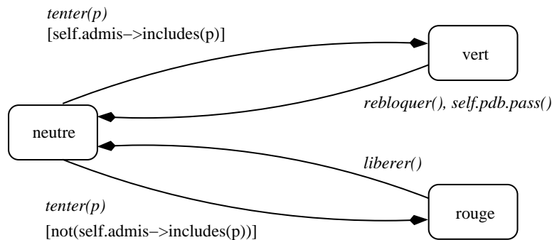
FIG. 6 – Diagramme d'état-transitions associé à la classe Porte .
