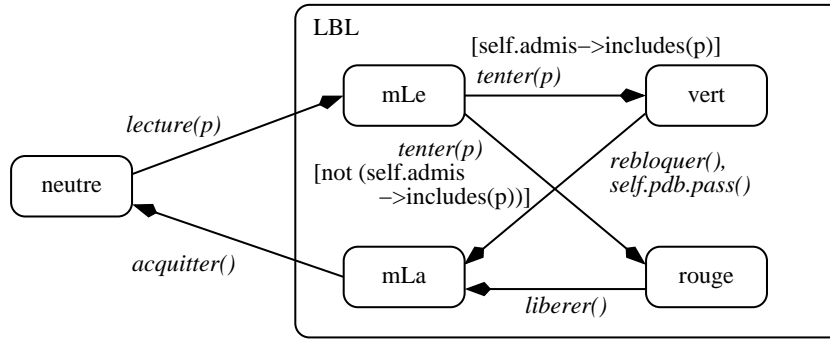
FIG. 8 – Diagramme d'état-transition du deuxième raffinement.
